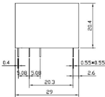
安装图
