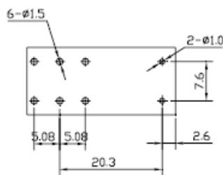
安装图
