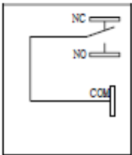
接线图(顶部)
